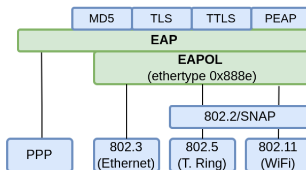
Figura 2.22: Capas del protocolo 802.1x
