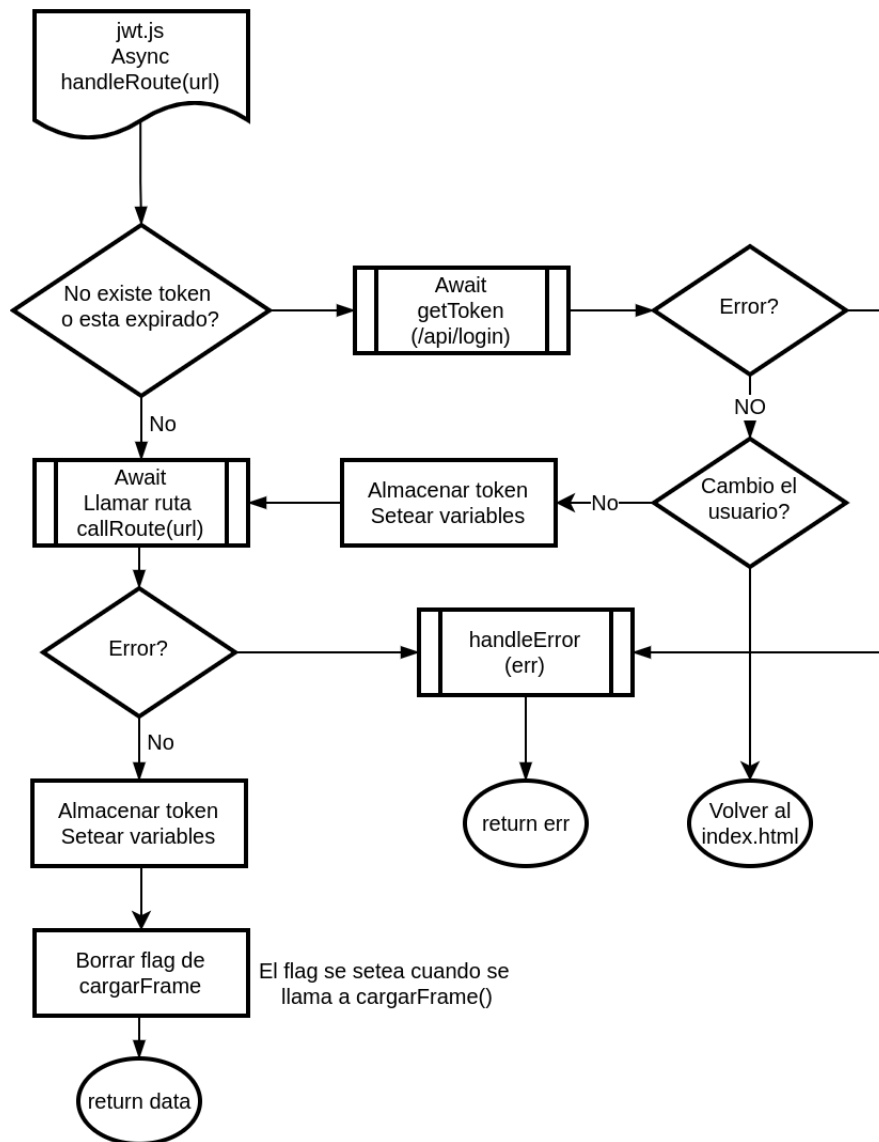
Figura 4.11: Diagrama de flujo para la función handleRoute()
