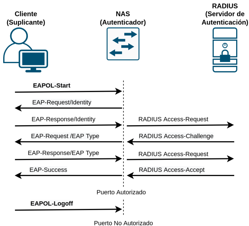
Figura 2.23: Flujo de mensajes 802.1x
