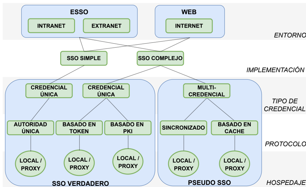
Figura 2.4: Taxonomía de los sistemas SSO
