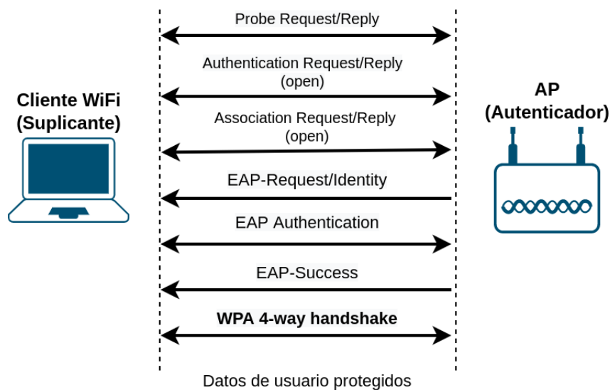
Figura 2.24: Autenticación WPA-Enterprise
