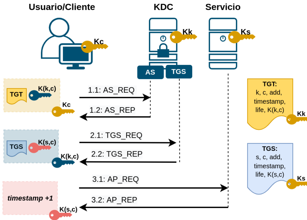
Figura 2.13: Intercambio de mensajes para Kerberos
