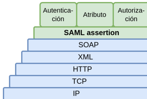
Figura 2.19: Stack de protocolos para SAML
