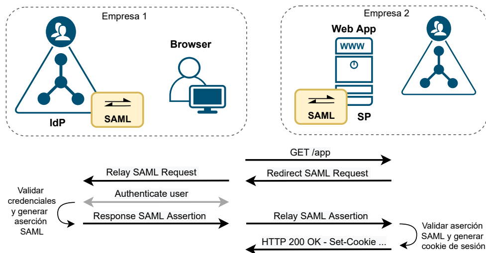
Figura 2.20: Flujo típico de mensajes SAML.
