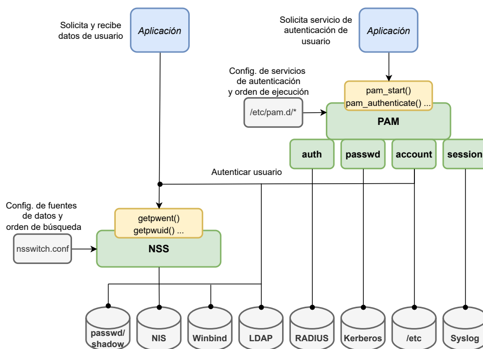
Figura 2.5: Autenticación en Linux
