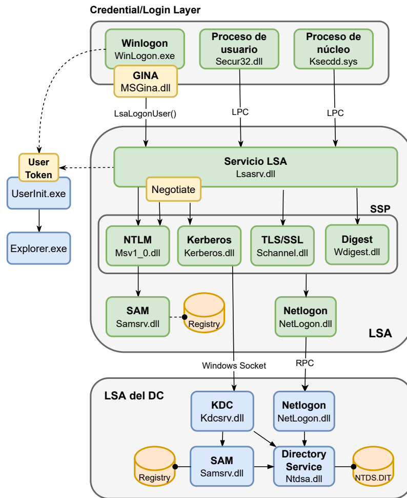
Figura 2.8: Autenticación en Windows
