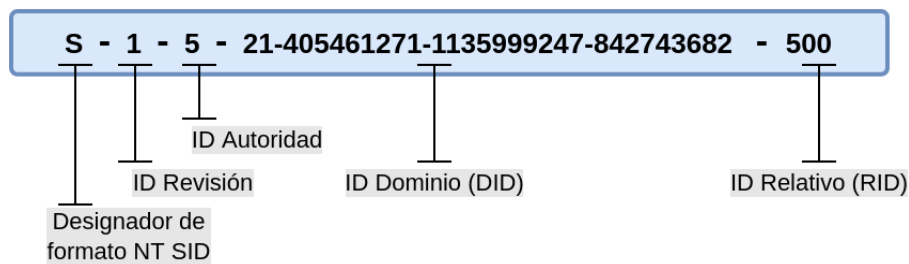
Figura 2.6: Formato de un SID
