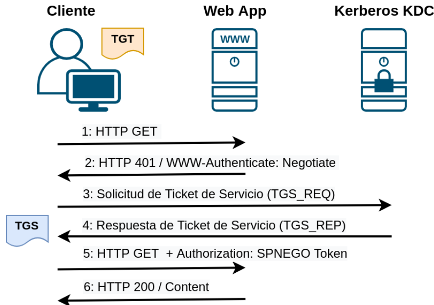
Figura 2.11: Autenticación HTTP utilizando SPNEGO
