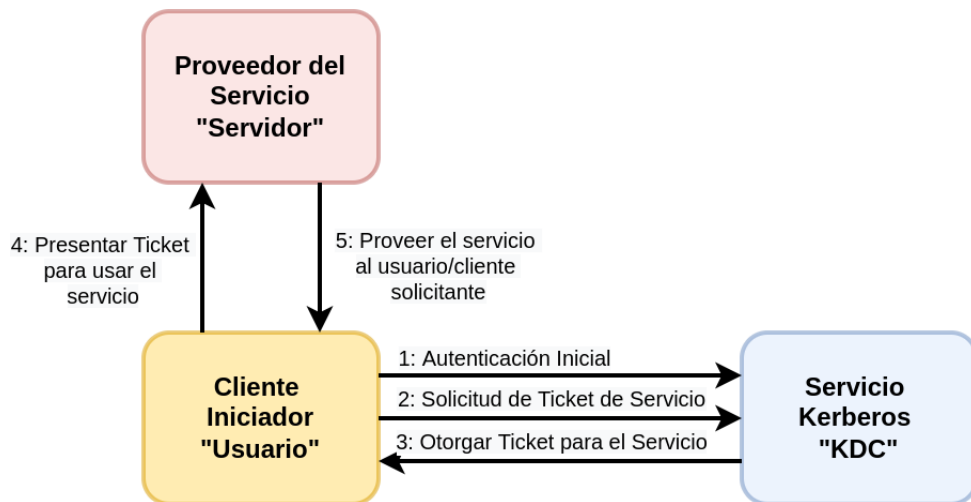
Figura 2.12: Esquema simplificado del modelo de autenticación de Kerberos
