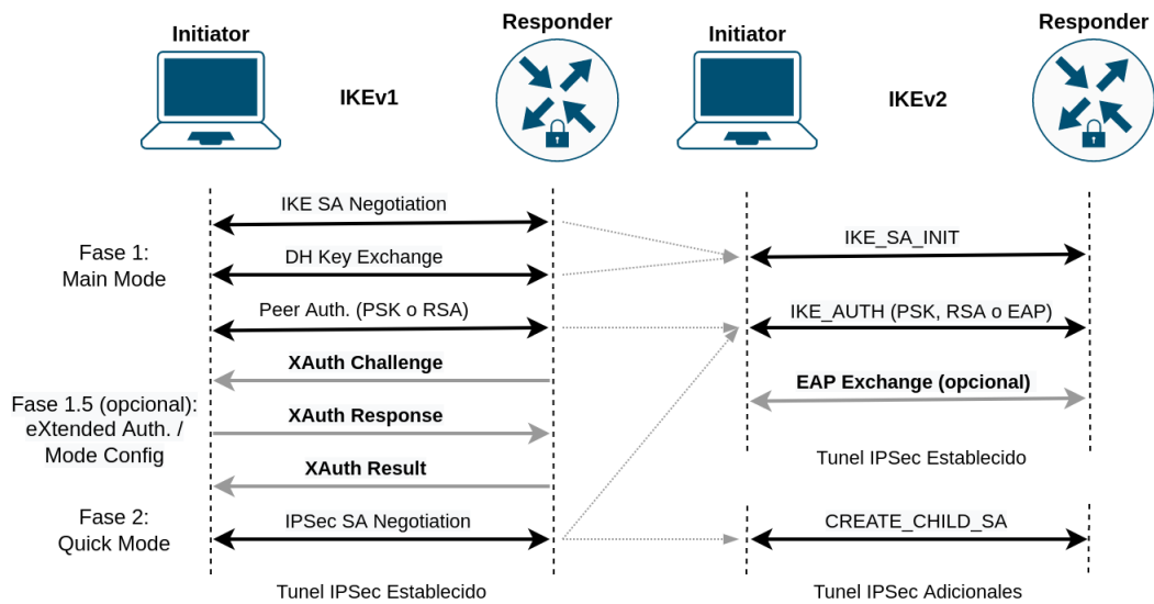
Figura 2.25: Autenticación en IKEv1 e IKEv2
