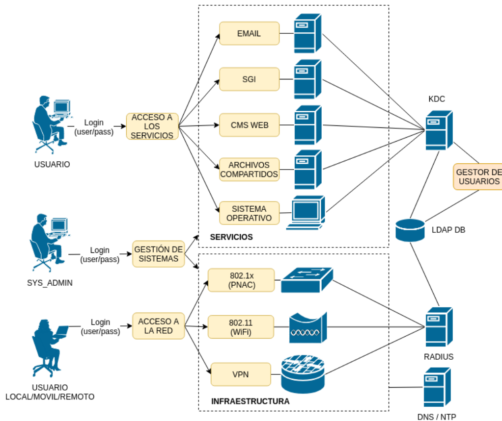
Figura 3.7: Esquema ilustrativo de la arquitectura de autenticación propuesta
