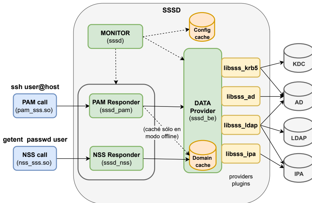
Figura 3.4: Arquitectura de SSSD
