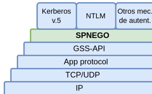
Figura 2.10: Pila de protocolos para SPNEGO
