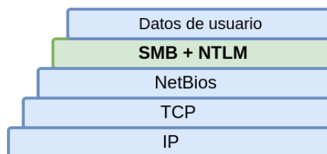
Figura 2.16: Capas del protocolo SMB
