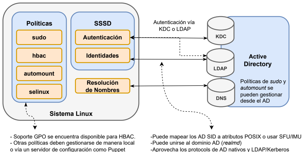
Figura 3.6: Integración directa de un cliente Linux a un servidor AD mediante SSSD
