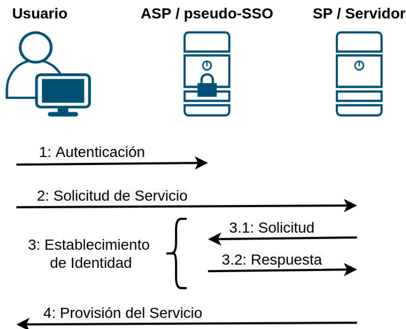
Figura 2.3: Flujo de mensajes en un sistema de autenticación SSO genérico
