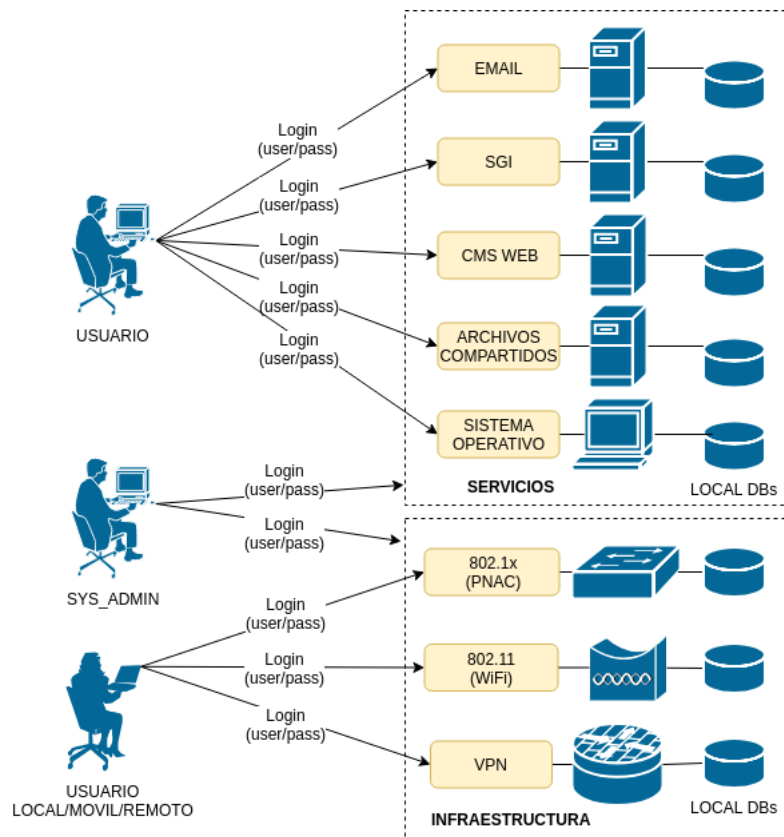
Figura 3.5: Esquema ilustrativo de los proceso de autenticación a los servicios e infraestructura del TEPM
