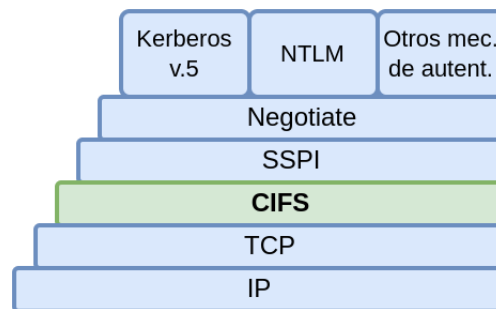
Figura 2.17: Capas del protocolo SMB/CIFS
