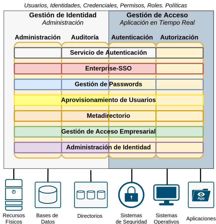
Figura 3.1: Visión general de un sistema de IAM
