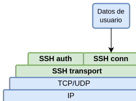
Figura 2.15: Capas del protocolo SSH
