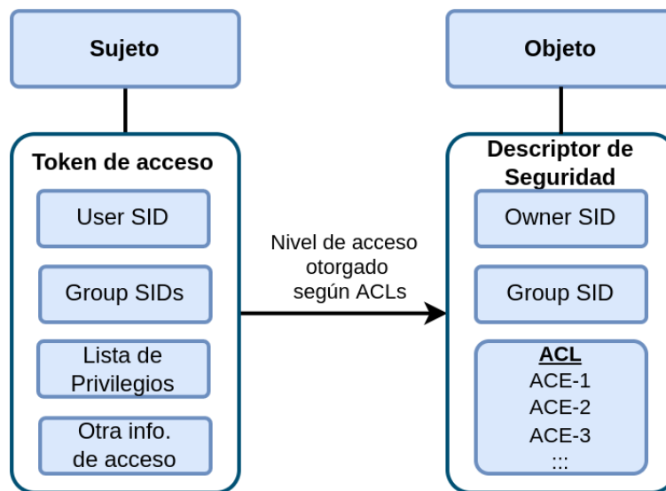
Figura 2.7: Autorización en Windows
